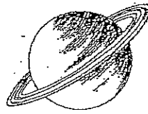
Uranus
